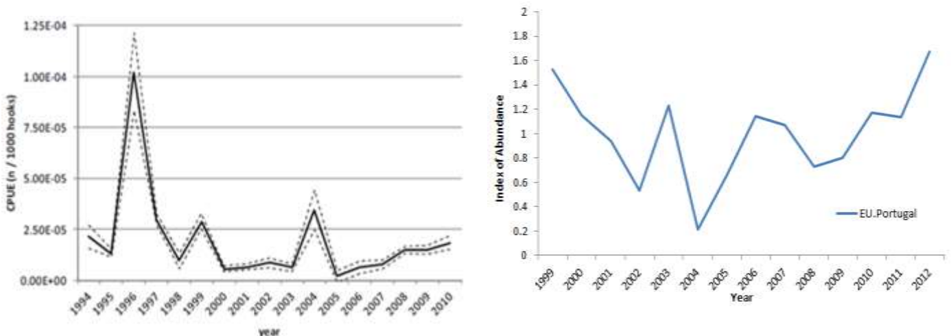
Fig. 2. Requin-taube bleu : Séries de PUE standardisées du requin-taube bleu capturé dans l'océan Indien par les flottilles japonaises (1994–2010, à gauche) et portugaises (1999–2012, à droite).
