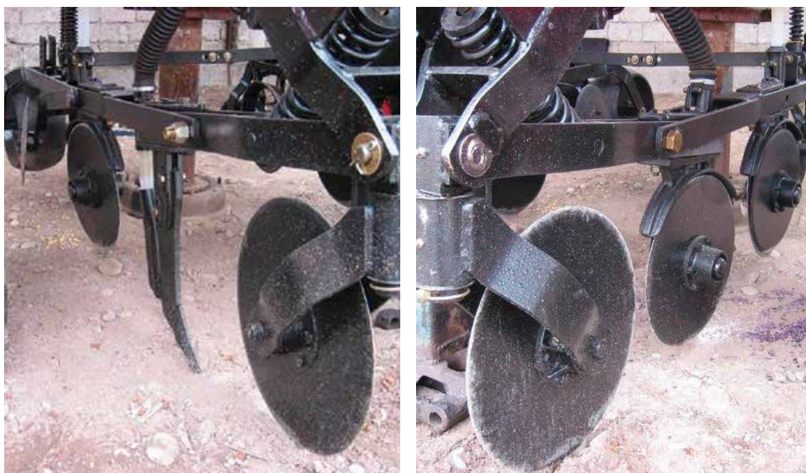
Рисунок 34. Долотовидный (слева) и двухдисковый (справа) сошники для внесения удобрений
