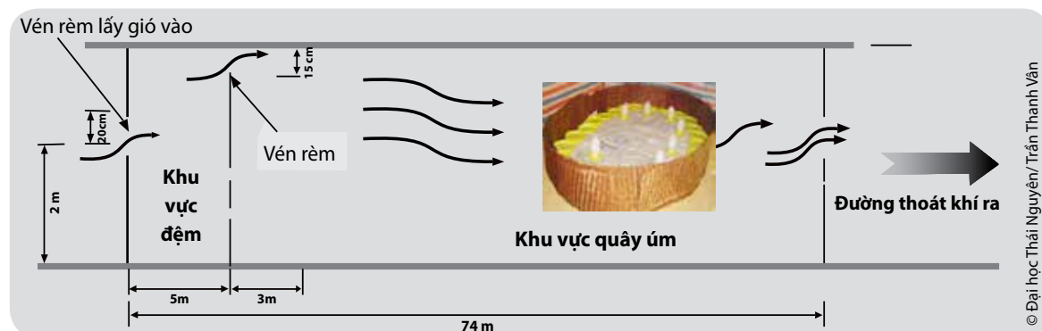
Hình 36. Cách tạo thông thoáng cho quây úm gà con
