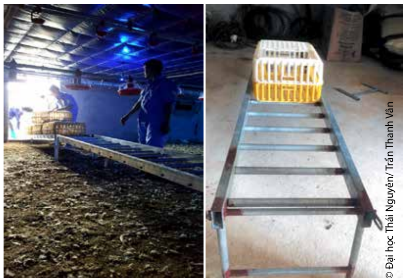
Hình 40. Lồng nhốt gà thịt và đường con lăn vận chuyển lồng gà từ chuồng ra ngoài
