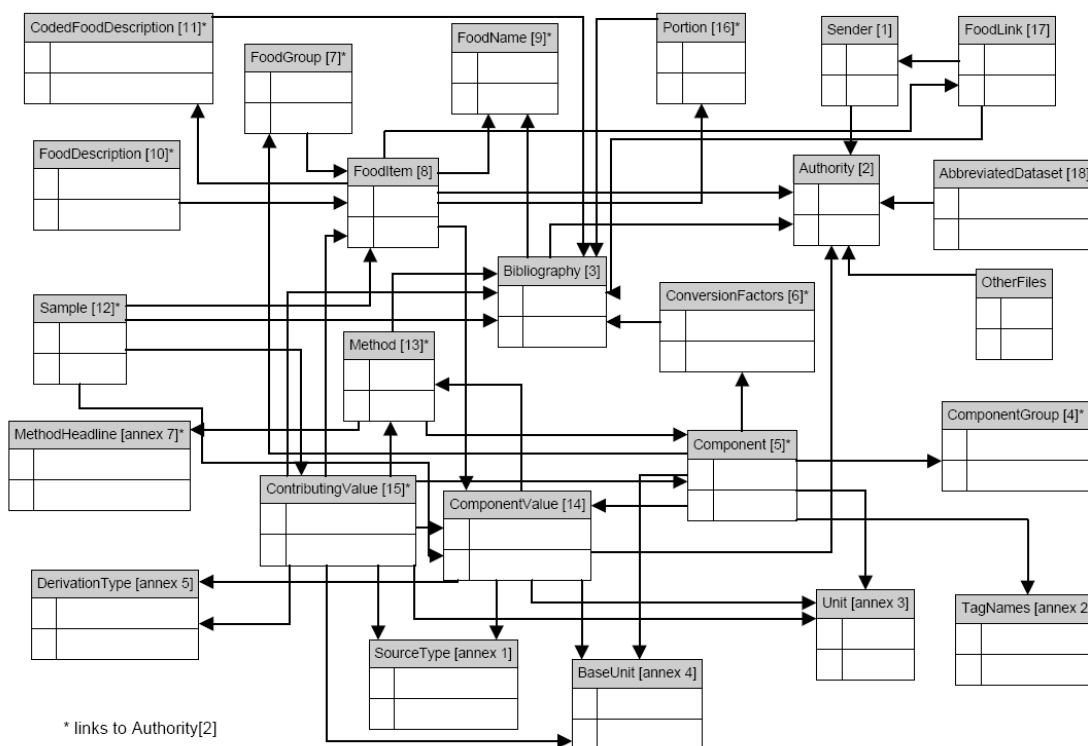
ER diagram
